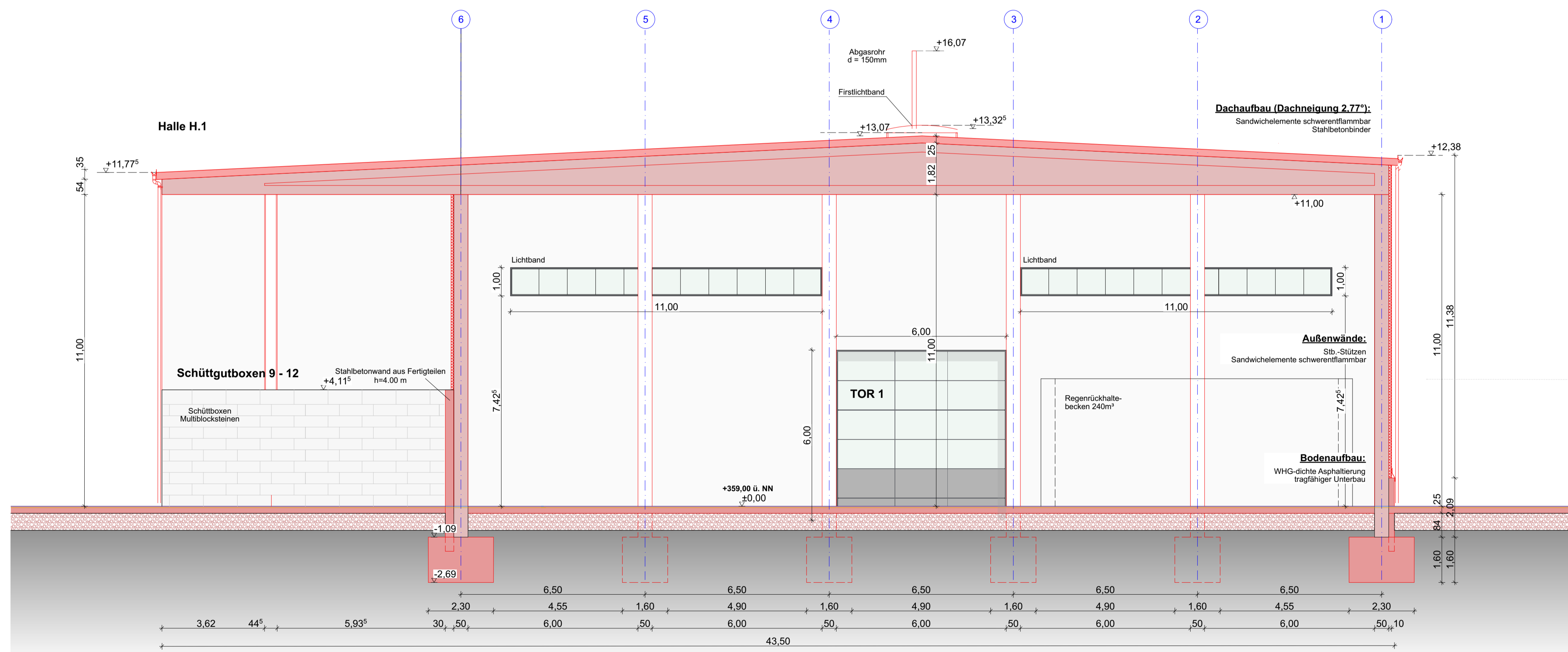
SCHNITT 2 - 2
